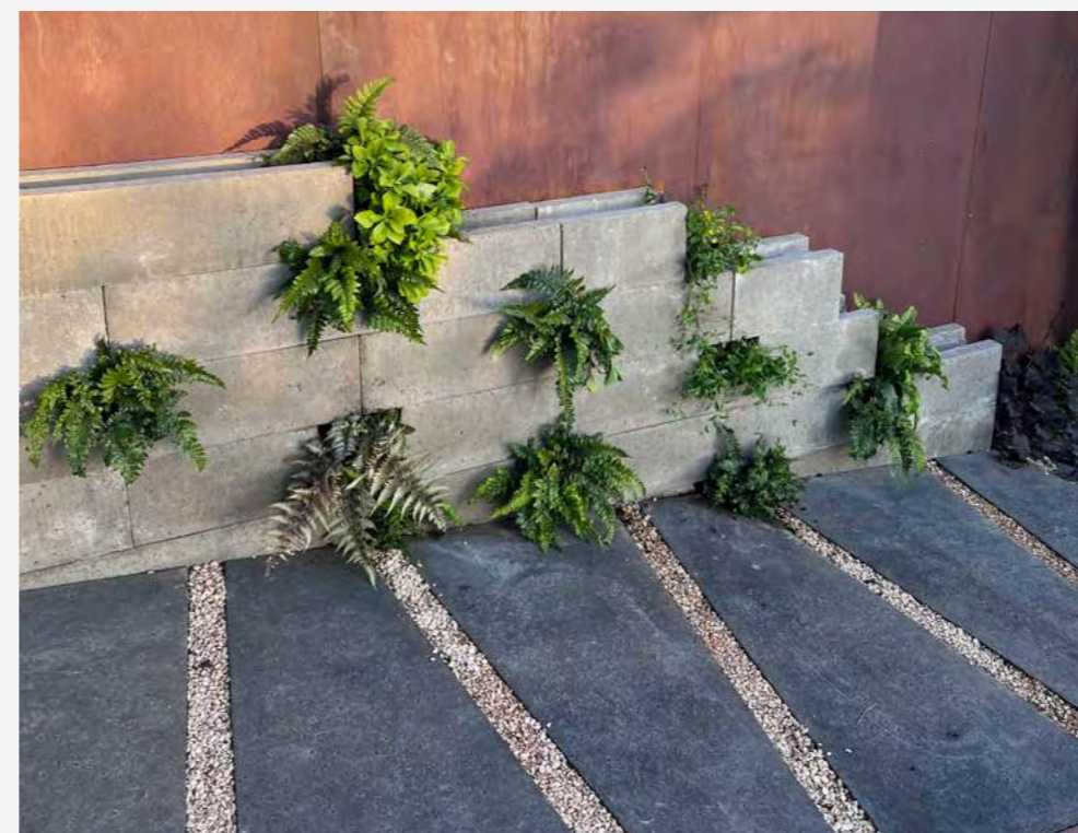
Projekt: Van den Heuvel Tuinen | Stapelelemente Grünwand und Stapelelement 100 x 20 x 20 cm - grau
