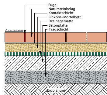
Systemskizze 3b (Schnittzeichnung) Aufbau Pflasterfläche
