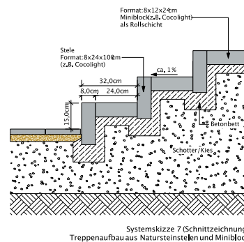
Stufenanlage aus Modulsteinen
