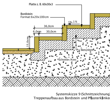
Stufenanlage aus Bordstein & Pflaster
