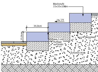
Stufenanlage aus Blockstufen
