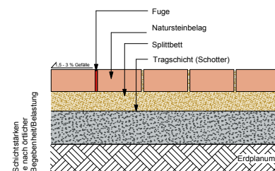
Systemskizze 3a (Schnittzeichnung) Aufbau Pflasterfläche
