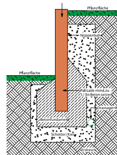
Versetzen von Palisaden und Modulsteinen
