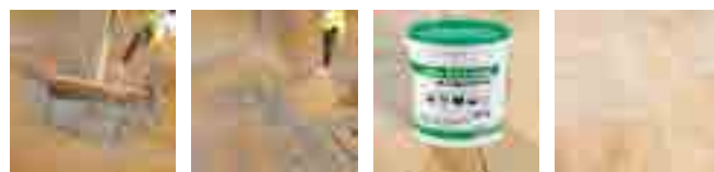
Mit Hartgummischieber und Wassersprühstrahl einschlänmen. Mit Wassersprühstrahl und feuchtem Besen reinigen. Mindestens 24 Stunden absperren und vor Regen schützen.
