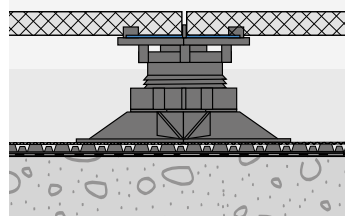
Verlegung mit Stelzlägern für Fliesen ab Stärke 20 mm
