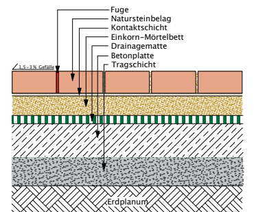
Systemskizze 3b (Schnittzeichnung) Aufbau Pflasterfläche
