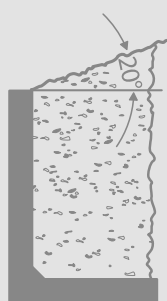
B | Böschung Geländeneigung 20^\circ , Verkehrslast bis p=\text{kN/m}^2
