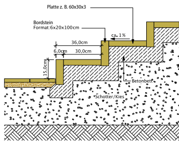
Systemskizze 9 (Schnittzeichnung) Treppenaufbau aus Bordstein und Pflasterklinker
