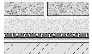
Verlegung im Kies-/Splittbett
