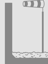
F | freistehende Wand mit Windlast bis q=0,65 \text{ kN/m}^2
