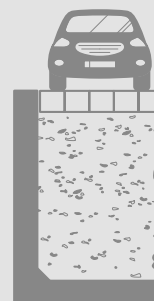
E | Verkehrslast bis p=5 \text{ kN/m}^2 , mit Verdichtungserddruck e_{\text{vh}}=25 \text{ kN/m}^2
