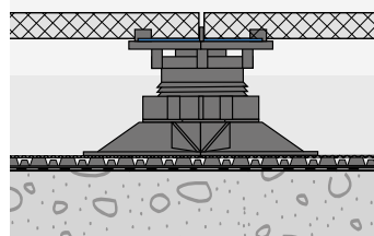
Verlegung mit Stelzlagnern für Fliesen ab Stärke 20 mm
