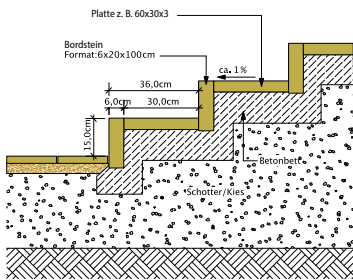
Stufenanlage aus Bordstein & Pflaster
