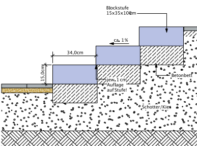
Stufenanlage aus Blockstufen
