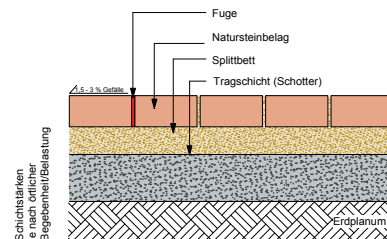
Systemskizze 3a (Schnittzeichnung) Aufbau Pflasterfläche
