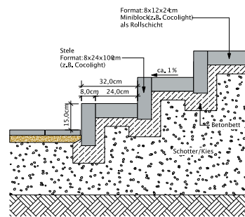
Stufenanlage aus Modulsteinen
