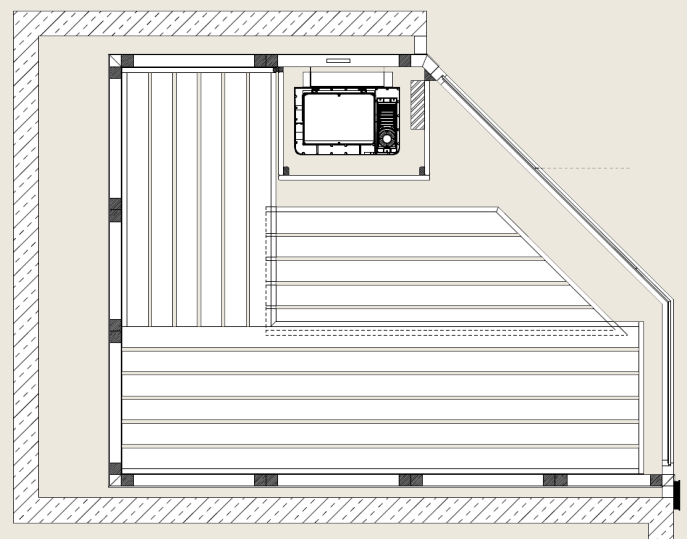
5-Eck / EckEinstieg 45°
