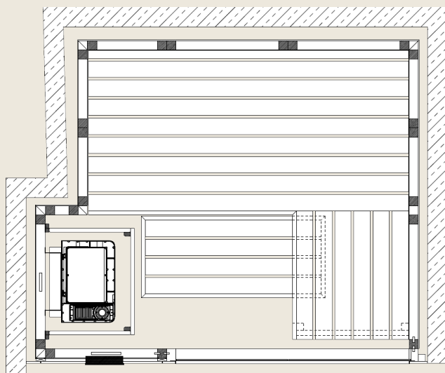
Aussparung
